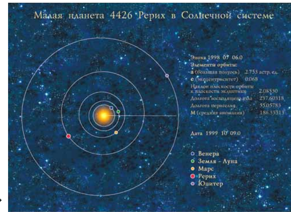
Схема орбиты малой планеты Roerich в Солнечной системе
